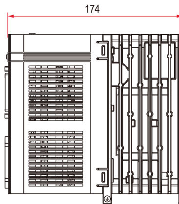
侧视图
