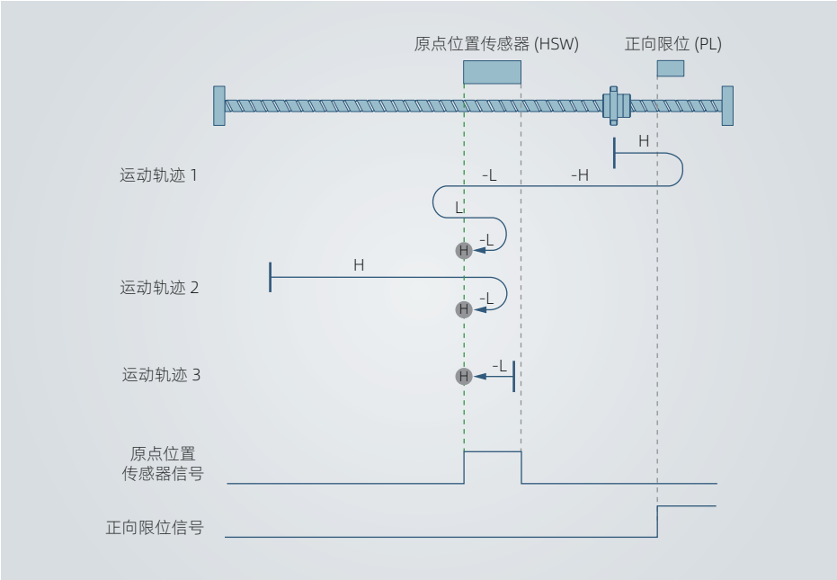
图 4-46 原点模式 23 轨迹及信号状态
