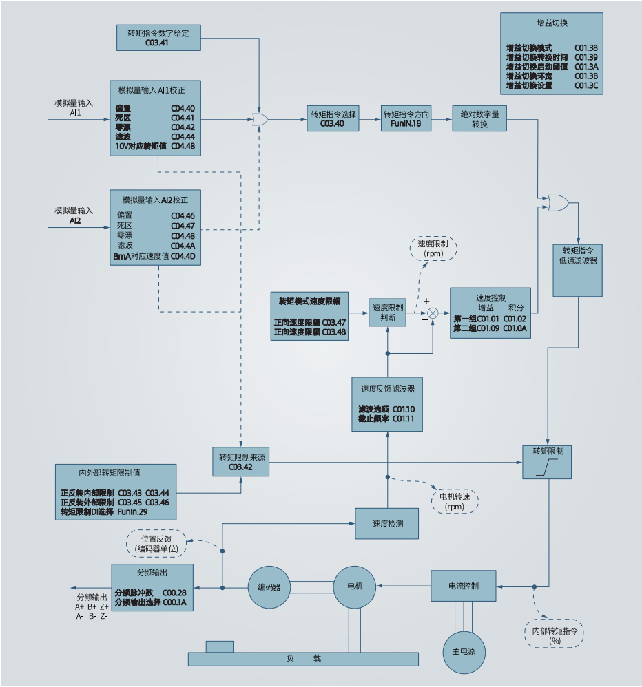
图 4-72 转矩控制模式功能框图
