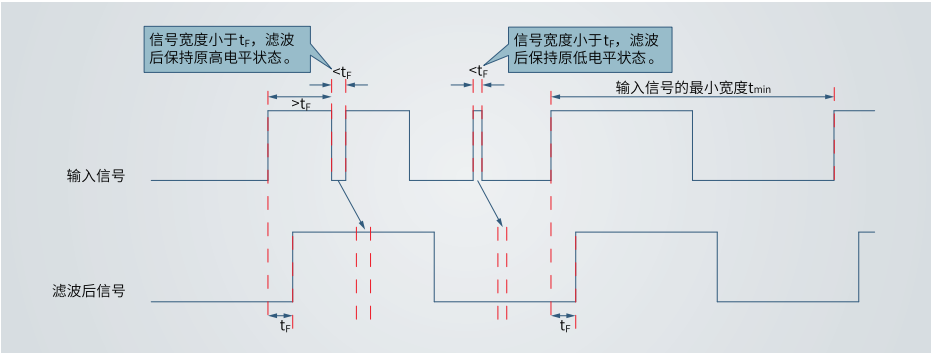
图 4-6 滤波信号波形示意图
