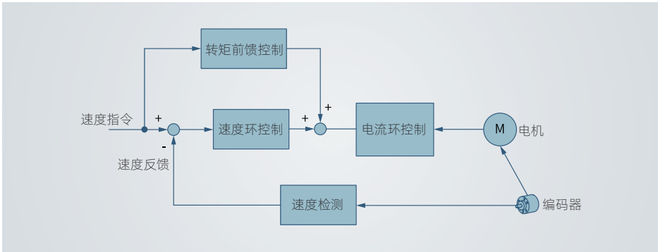
图 7-1 转矩前馈控制框图
