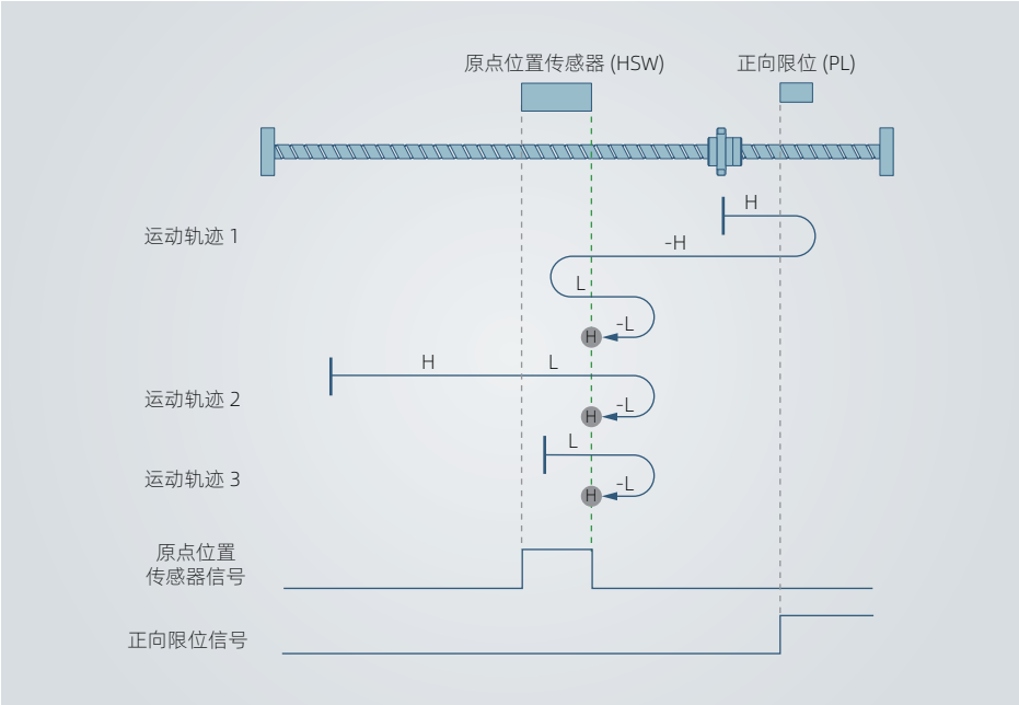
图 4-48 原点模式 25 轨迹及信号状态
