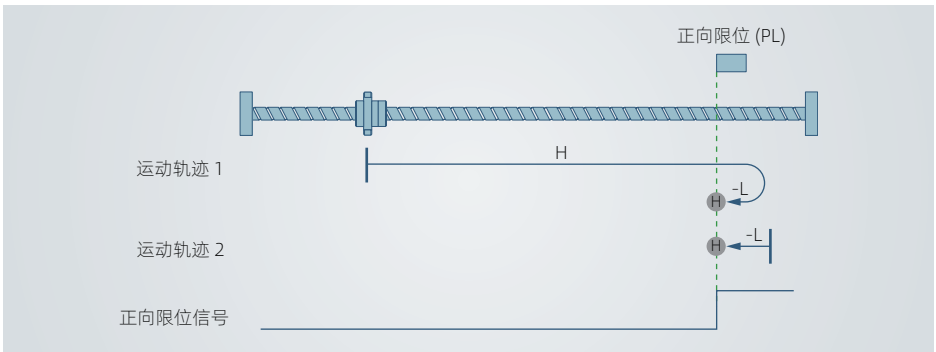
图 4-41 原点模式 18 轨迹及信号状态
