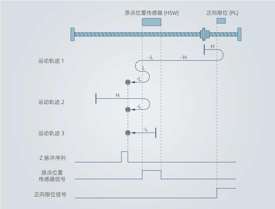
图 4-32 原点模式 7 轨迹及信号状态
