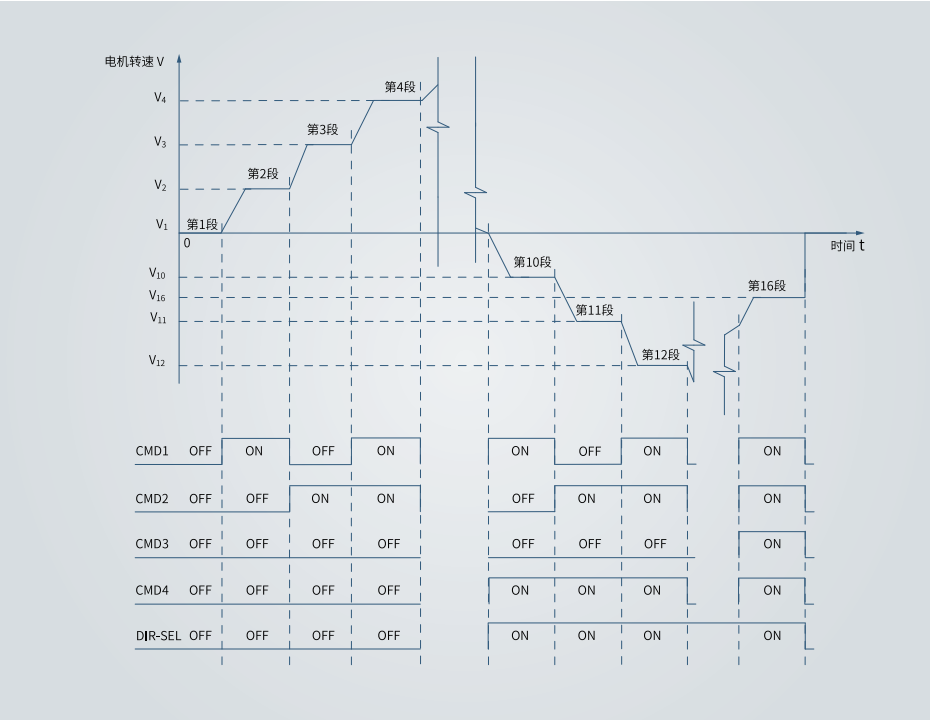
图 4-63 多段速度曲线举例
