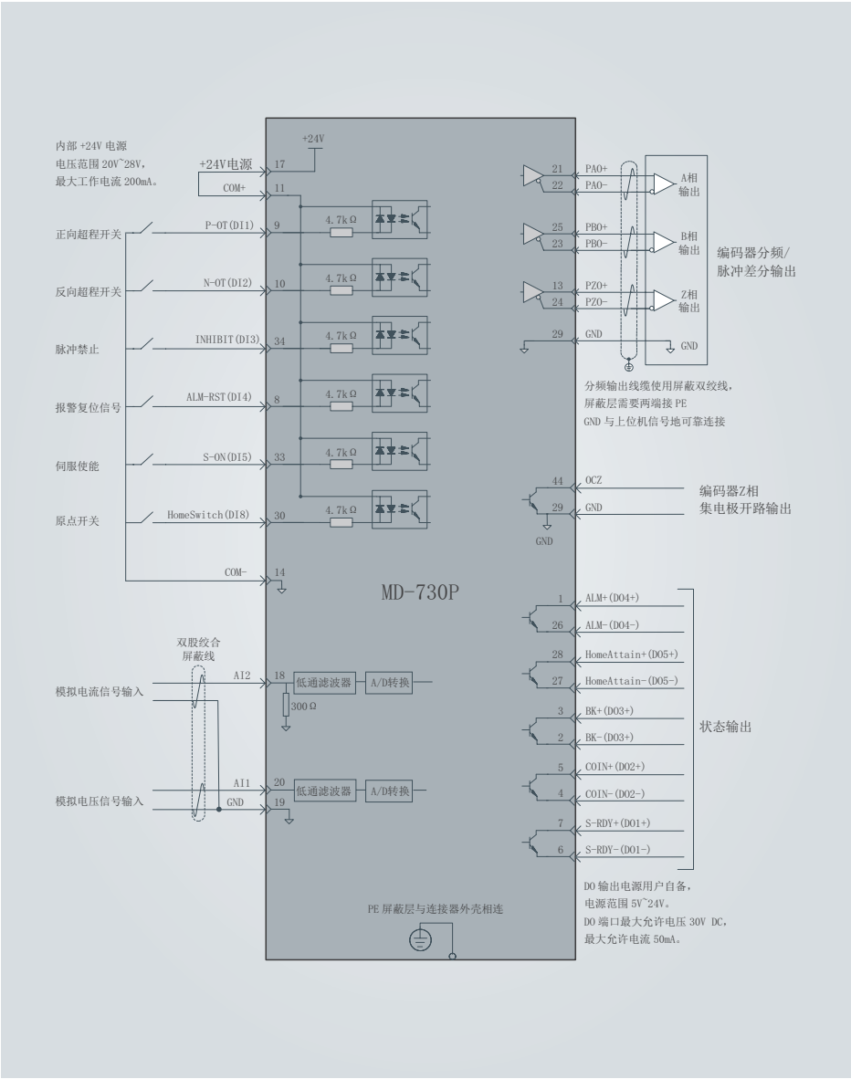
图 3-2 转矩模式接线示意图
