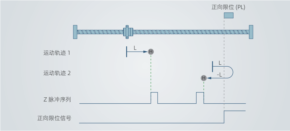
图 4-55 原点模式 34 轨迹及信号状态
