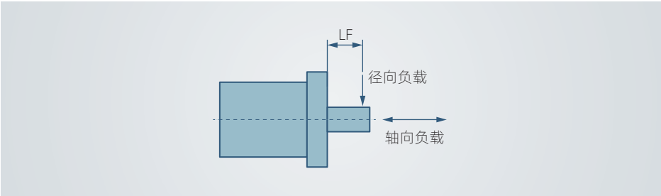
图 9-6 电机径向及轴向载荷示意图
