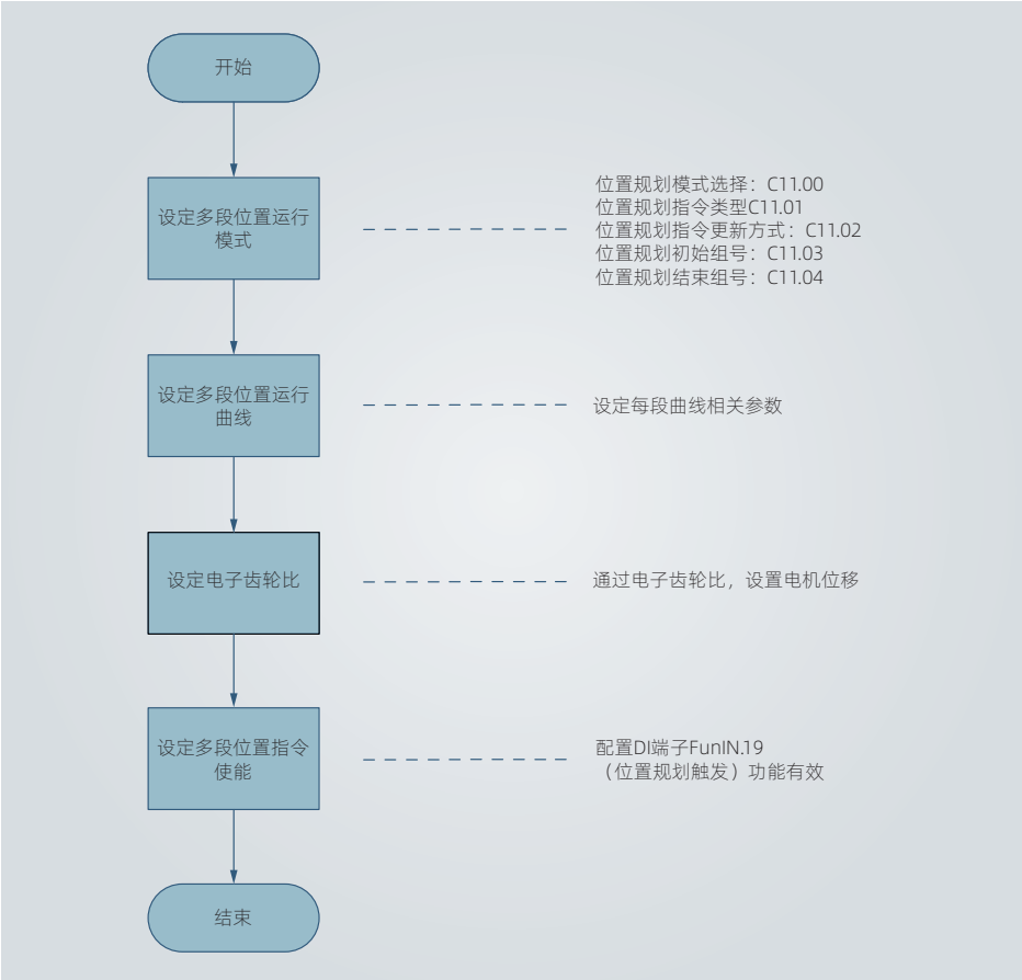
图 4-7 多段位置指令来源设置流程
