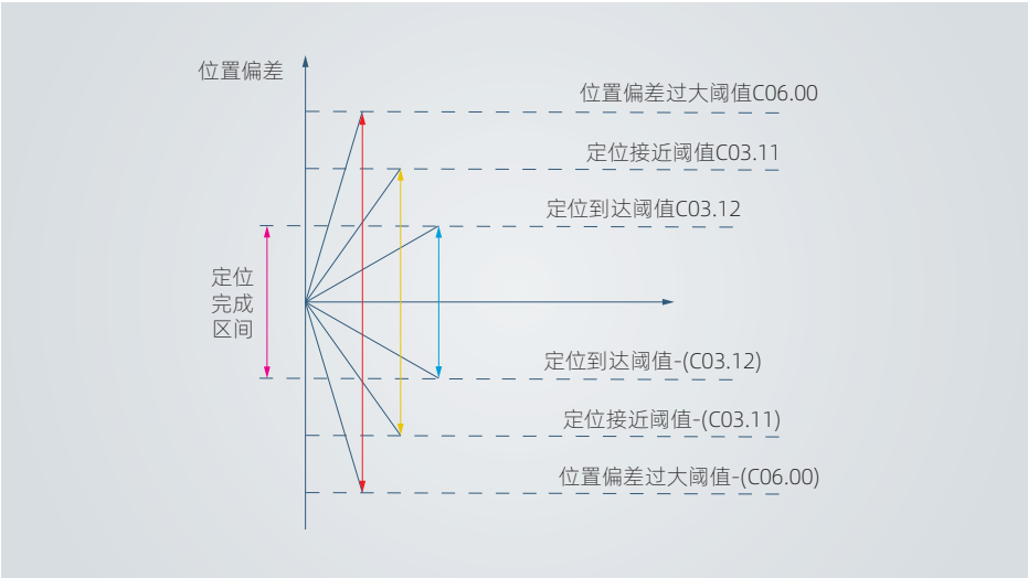
图 4-19 位置偏差相关信号
