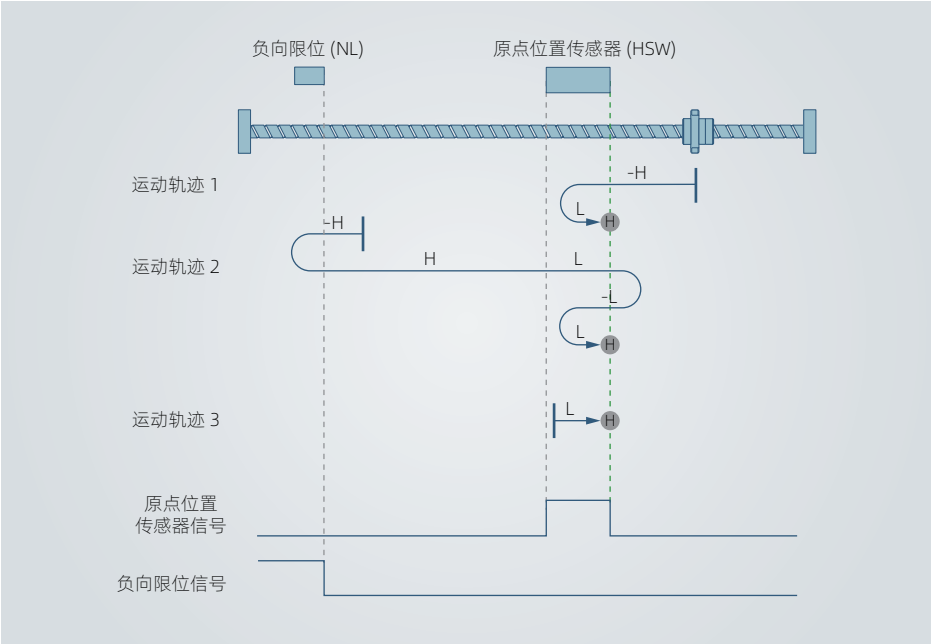
图 4-50 原点模式 27 轨迹及信号状态
