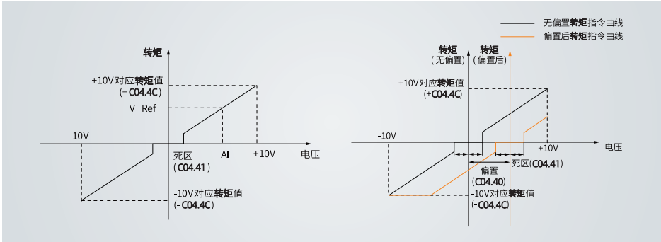
图 4-77 无偏置 AI1 示意图 (左) & 偏置后 AI1 示意图 (右)
