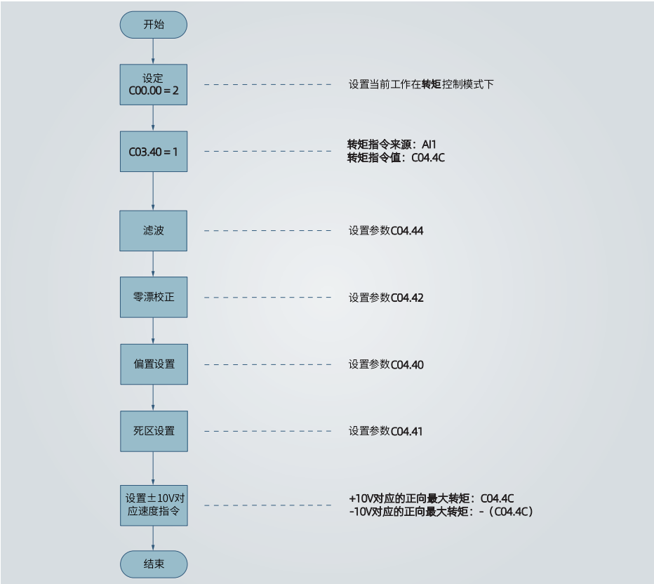
图 4-74 模拟量电压转矩指令操作流程
