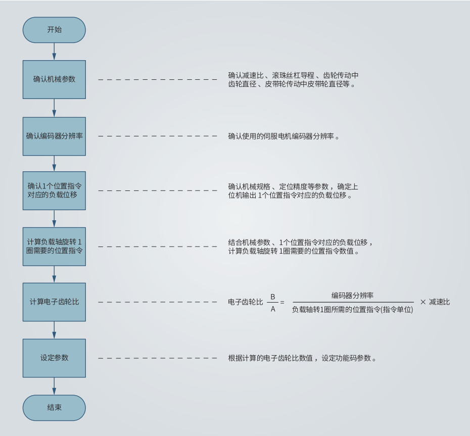
图 4-13 电子齿轮比设定步骤
