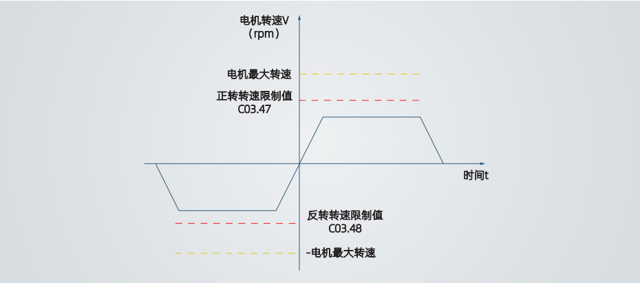
图 4-89 速度限制曲线图
