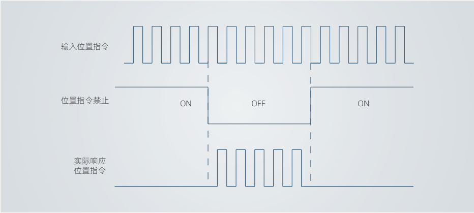
图 4-12 位置指令禁止功能波形举例
