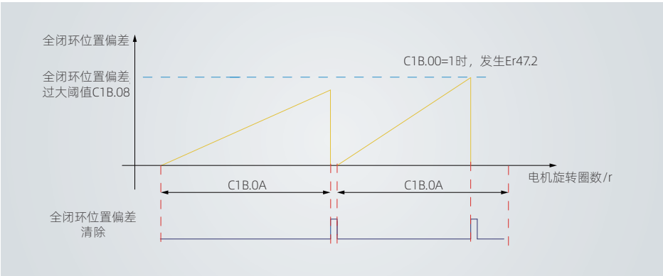
图 4-92 全闭环位置偏差清除说明
