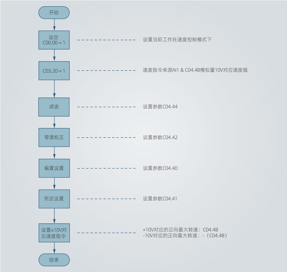
图 4-58 模拟量电压速度指令操作流程图
