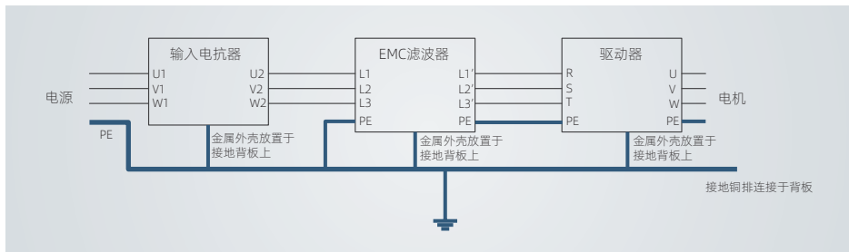
图 12-1 电抗器安装方式示意图
