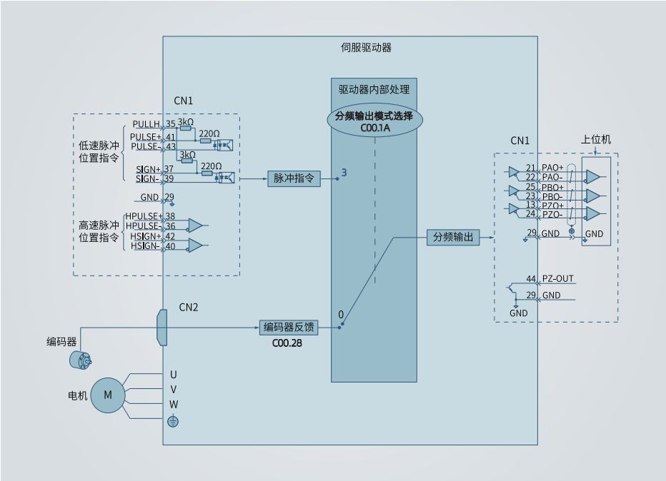
图 4-17 分频输出原理示意图
