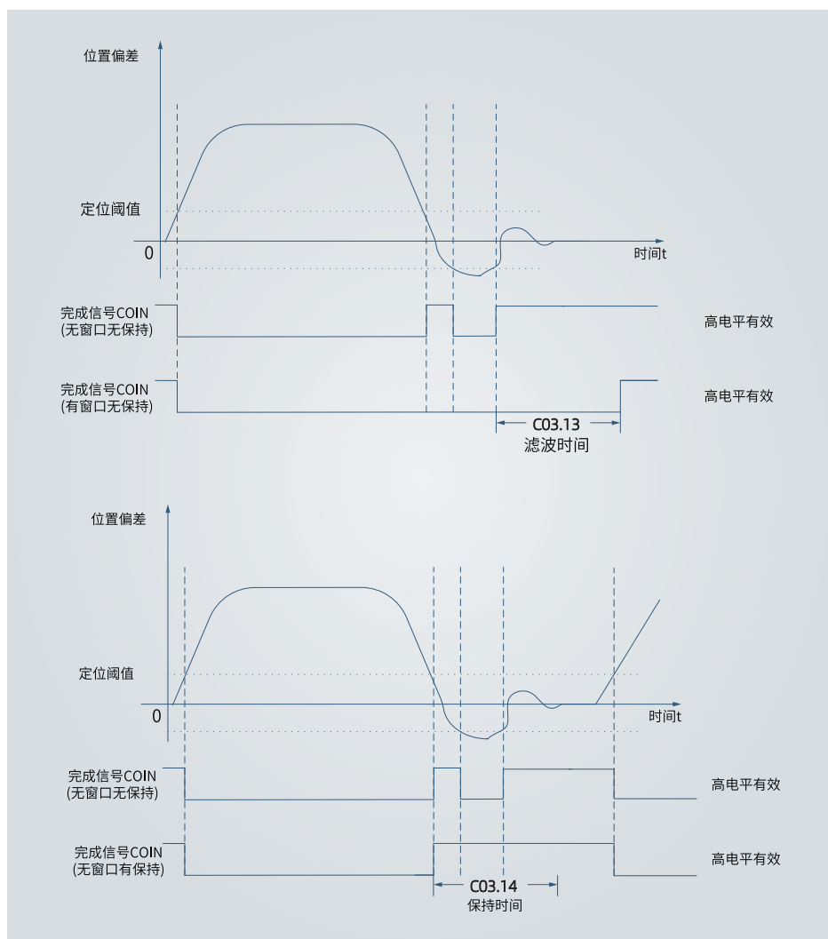
图 4-20 定位完成窗口时间和保持时间的原理图
