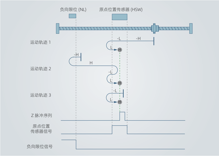
图 4-38 原点模式 13 轨迹及信号状态
