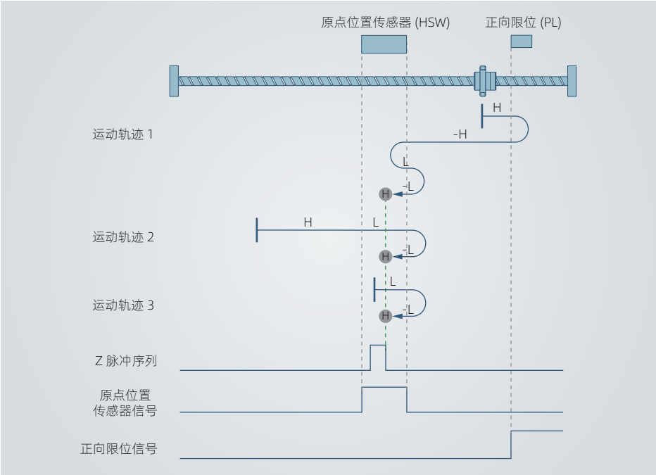
图 4-34 原点模式 9 轨迹及信号状态
