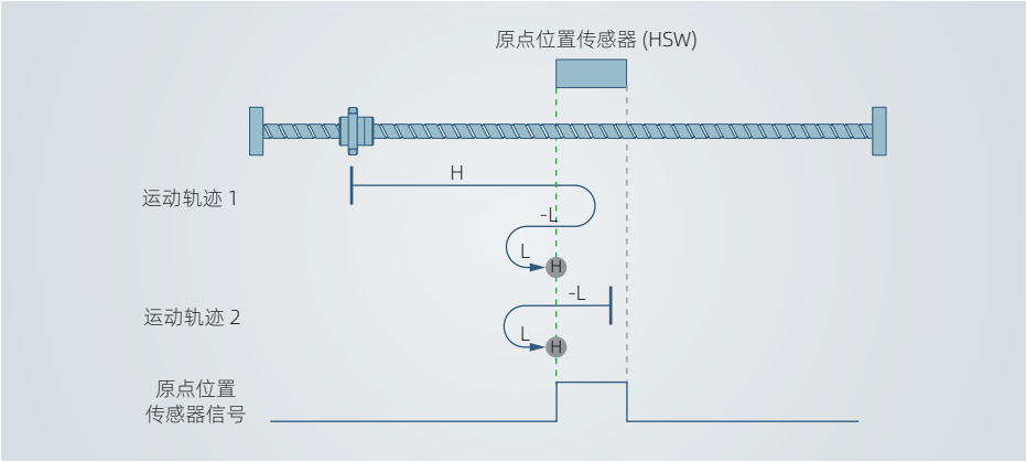
图 4-43 原点模式 20 轨迹及信号状态
