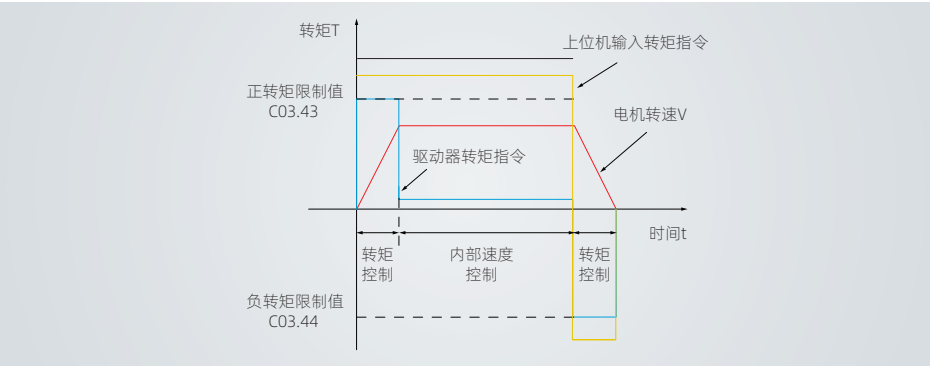
图 4-83 C03.42=0 转矩限制曲线
