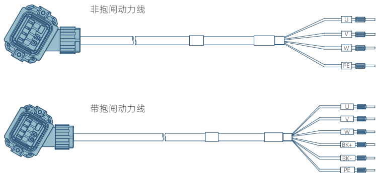
图 3-4 端子型电动力线缆示意图
