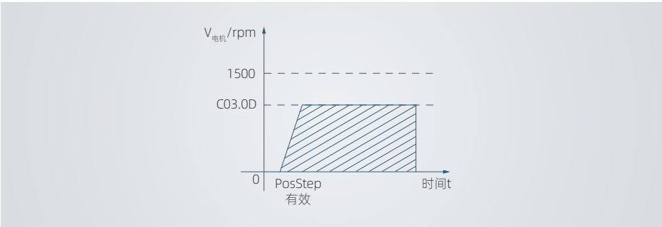
图 4-11 C03.00=2 时，电机运行曲线
