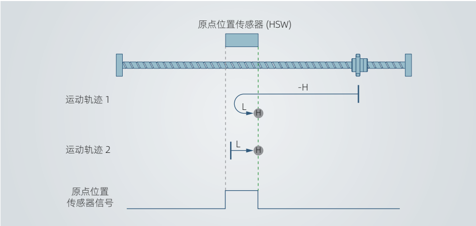
图 4-44 原点模式 21 轨迹及信号状态
