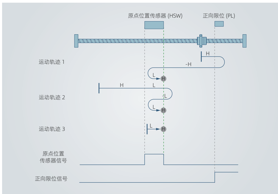
图 4-49 原点模式 26 轨迹及信号状态
