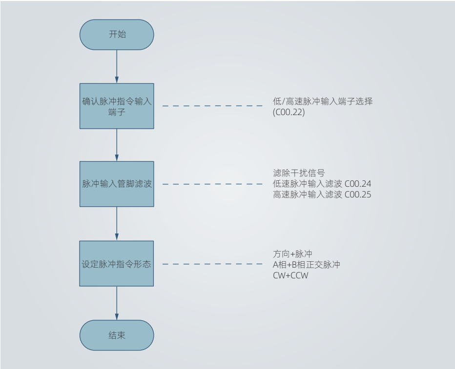
图 4-5 脉冲指令来源设置流程
