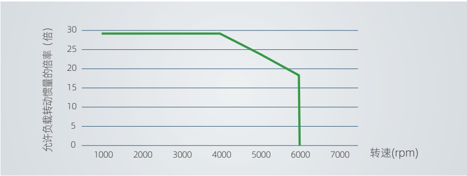
图 9-5 转速对应允许负载转动惯量的倍率
