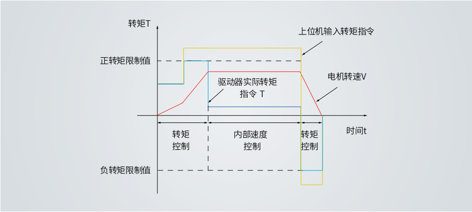
图 4-80 转矩给定与转矩限制
