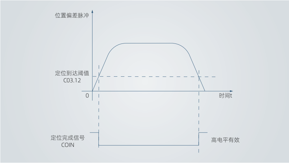
图 4-18 定位完成 / 接近功能说明
