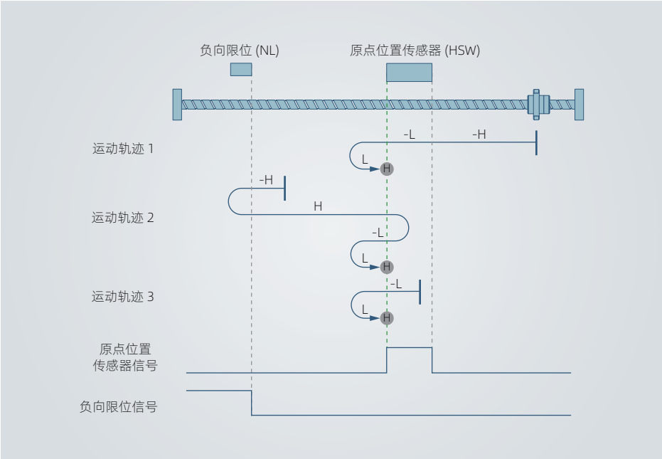
图 4-52 原点模式 29 轨迹及信号状态
