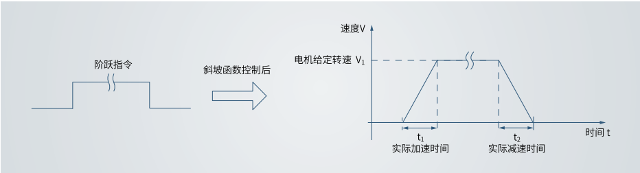
图 4-65 斜坡函数定义示意图
