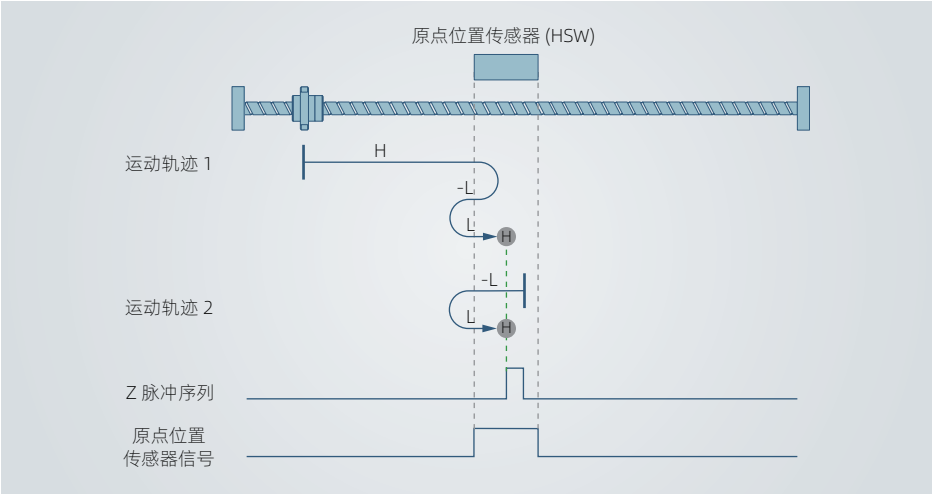
图 4-29 原点模式 4 轨迹及信号状态
