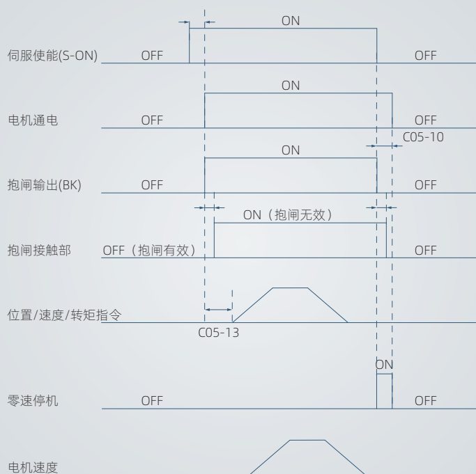
图 5-2 电机旋转时抱闸时序图
