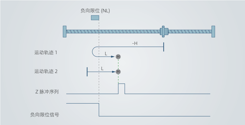
图 4-26 原点模式 1 轨迹及信号状态示意图
