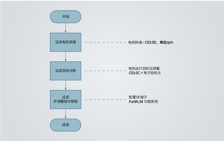
图 4-10 步进量指令来源设置流程
