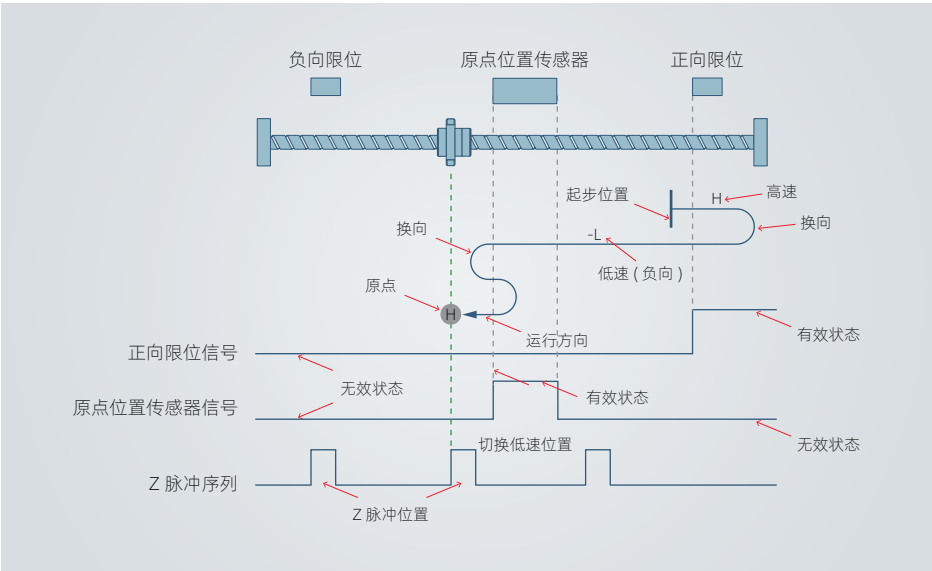
图 4-23 原点模式各图标含义示意图
