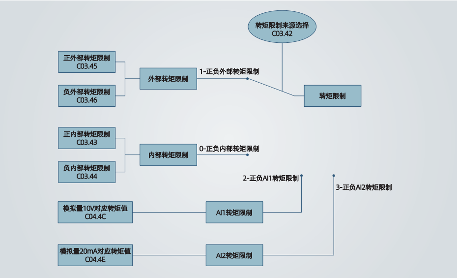
图 4-82 转矩限制来源
