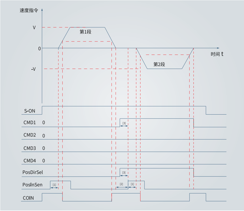
图 4-8 多段位置时序图
