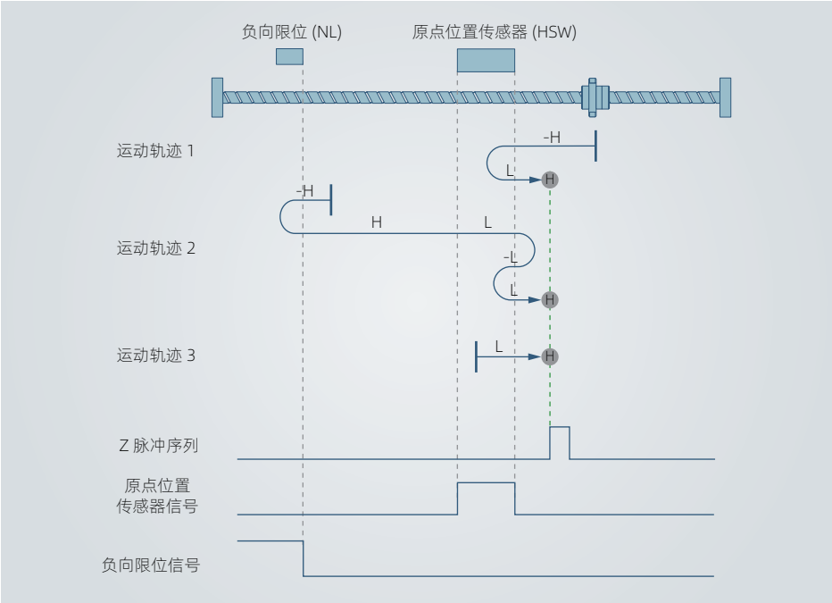
图 4-36 原点模式 11 轨迹及信号状态
