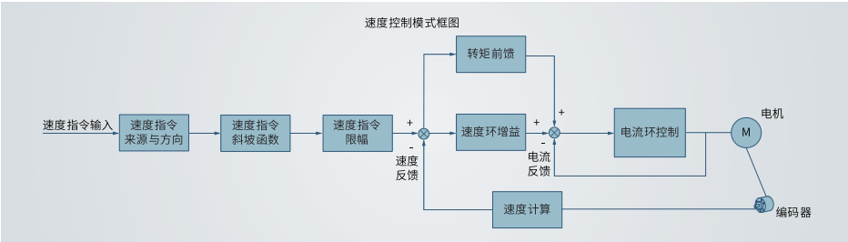
图 4-56 速度控制框图
